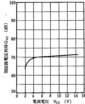
G_{VO} - V_{CC}
