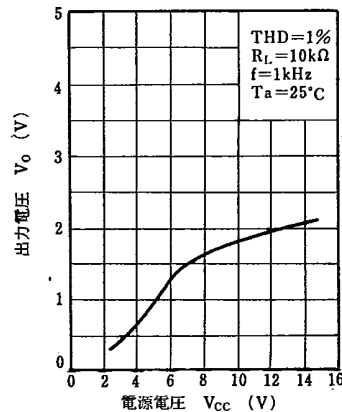
V_O - V_{CC}
