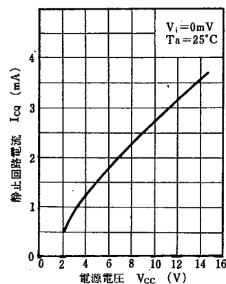
I_{CQ} - V_{CC}
